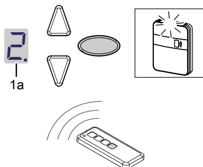
Fig. 10: Programmation de la fonction éclairage pour l'émetteur portatif
