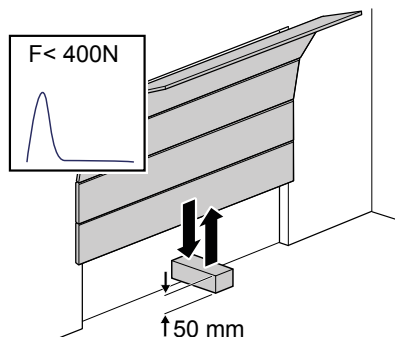
Fig. 12: Contrôle de la limitation d'effort
